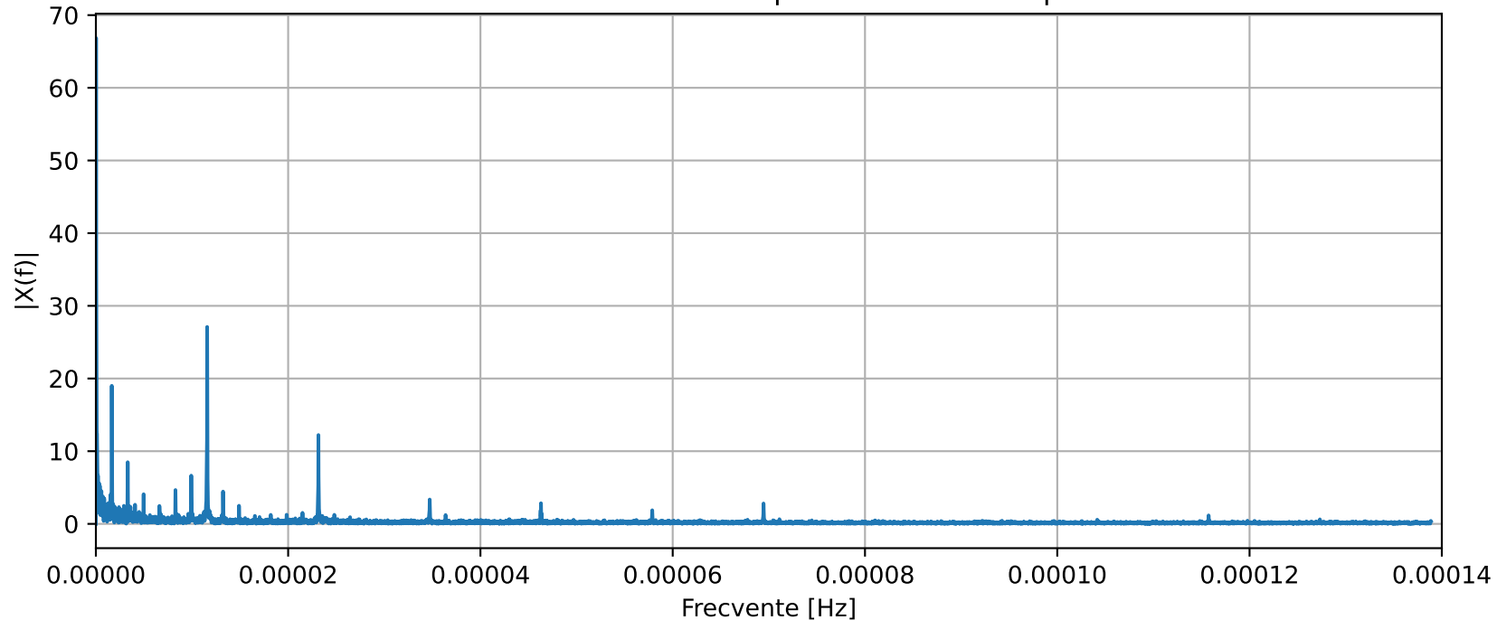
Transformata Fourier a semnalului dupa eliminarea componentei continue
